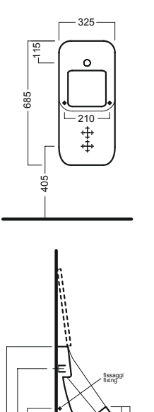
orinatoio sospeso con coperchio wall hung urinal with cover
