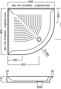
piatto doccia 90x90 angolare corner showertray 90x90
