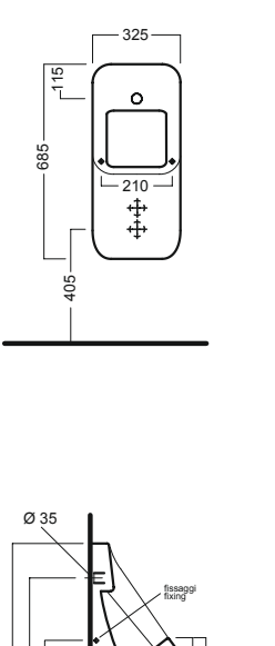
orinatoio sospeso wall hung urinal
