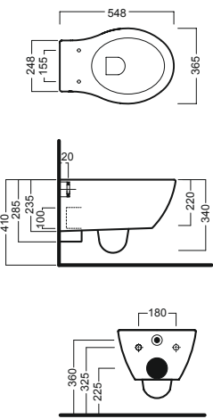
vaso sospeso wall hung wc
