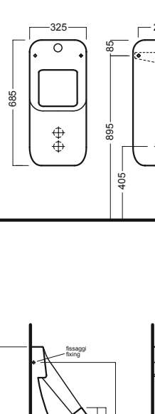
orinatoio sospeso con fotocellula wall hung urinal with photocell
