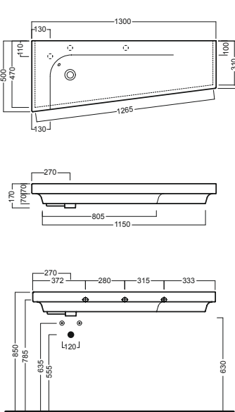
G-130 T destro G-130 T right
