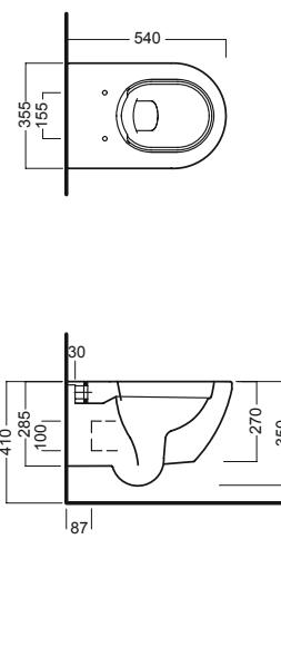
vaso sospeso rimless rimless wall hung wc
