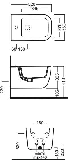
bidet sospeso wall hung bidet
