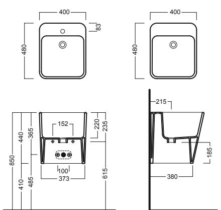
lavabo pilozzo sospeso wall hung sink
