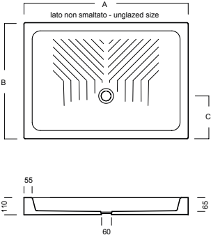
piatti doccia rettangolari rectangular showertrays
