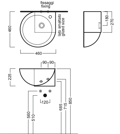
lavabo 46 sinistro washbasin 92 left
