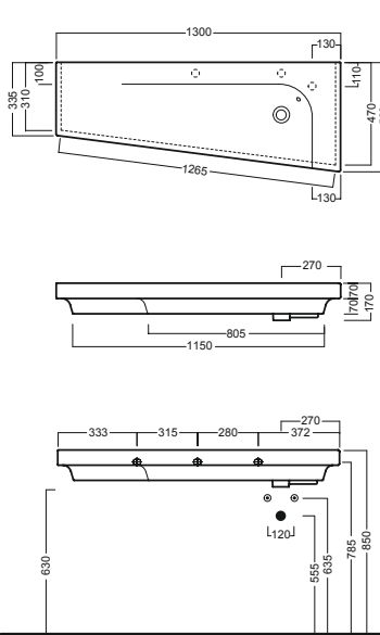
G-130 T sinistro G-130 T left
