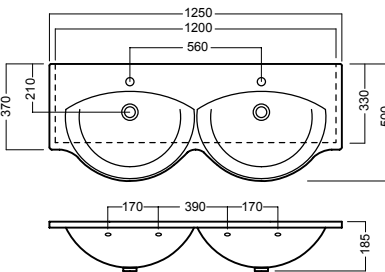
lavabo doppio 125 double washbasin 125
