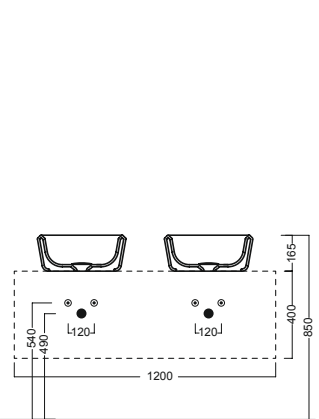
SLIDING wood system taglio 4 doppio - cut 4 double
