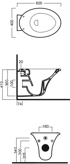
vaso sospeso wall hung wc
