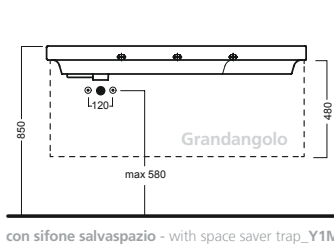
con sifone salvapazio - with space saver trap_Y1M5
