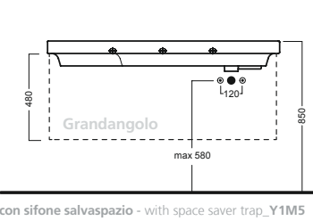
con sifone salvapazio - with space saver trap_Y1M5
