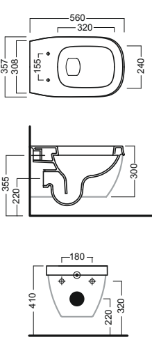
vaso sospeso wall hung wc
