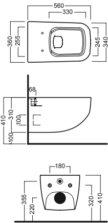
vaso sospeso rimless rimless wall-hung wc
