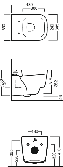
vaso sospeso wall hung wc
