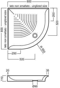
piatto doccia 80x80 angolare corner showertray 80x80
