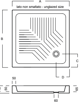
piatti doccia quadrati square showertrays
