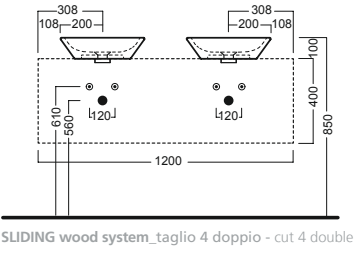
SLIDING wood system_taglio 4 doppio - cut 4 double
