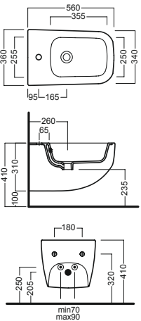
bidet sospeso wall-hung bidet
