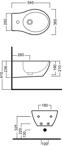
bidet sospeso wall hung bidet
