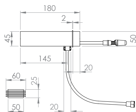
Vaso Sospeso Wall-hung WC
