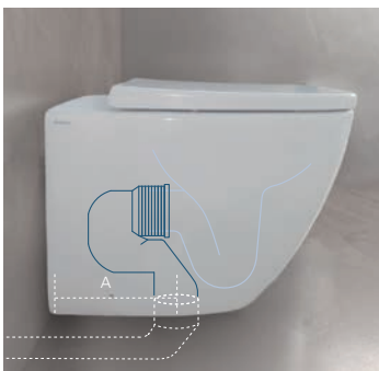
Bianca Vaso scarico universale traslato filo muro Bianca shifted universal outlet back to wall wc
