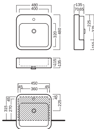
Apertura per installazione su piano Hole for surface installation
