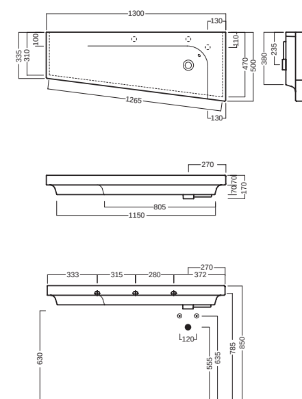
G-130 T sinistro G-130 T left
