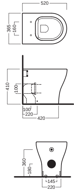
vaso filo muro PURE RIM PURE RIM back to wall wc
