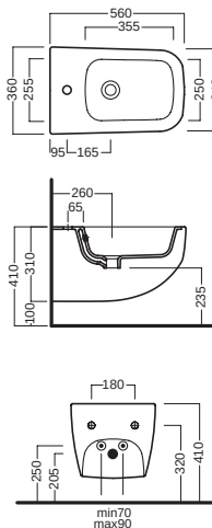
bidet sospeso wall-hung bidet
