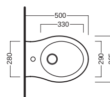
bidet filo muro_50 back to wall bidet_50
