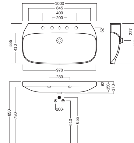
lavabo 100 washbasin 100
