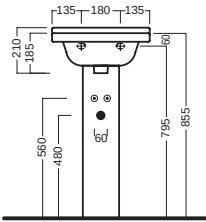
colonna_pedestal
