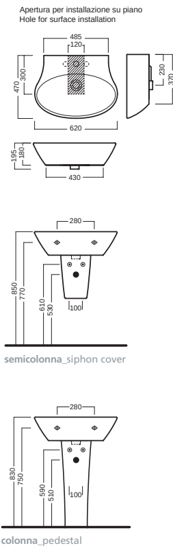
lavabo 62 washbasin 62
