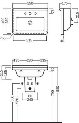
semicolonna_siphon cover
