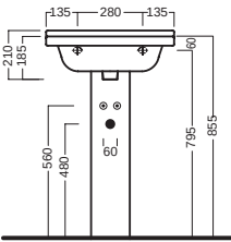
colonna_pedestal
