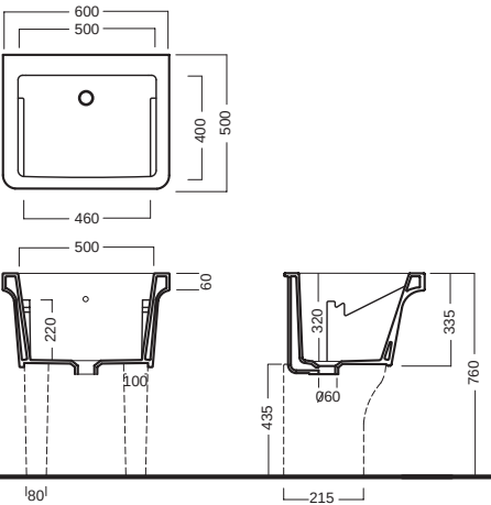
lavatoio 60 sink 60
