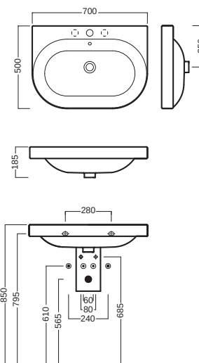
lavabo 70 washbasin 70
