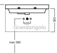
con sifone salvaspazio - with space saver trap_Y1M5
