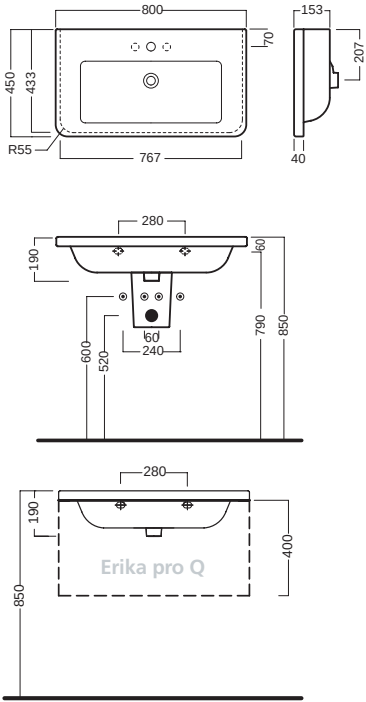
lavabo 80 washbasin 80
