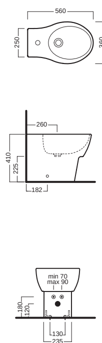
bidet filo muro back to wall bidet
