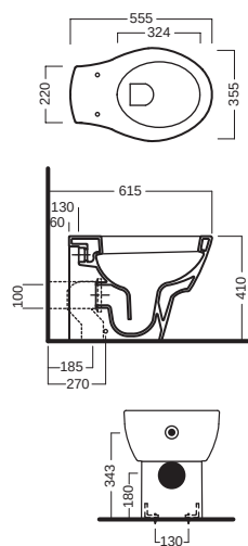
vaso wc
