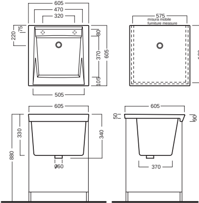
lavatoio 60 sink 60
