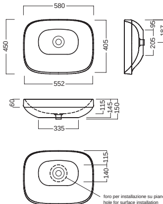
lavabo 80 washbasin 80
