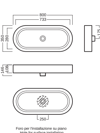
lavabo 80x35 washbasin 80x35
