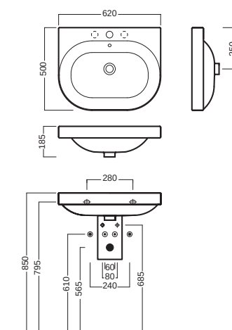
lavabo 62 washbasin 62
