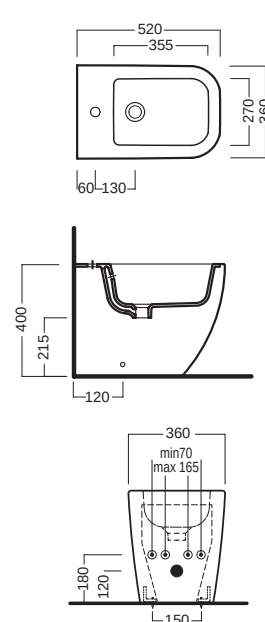
bidet filo muro back to wall bidet
