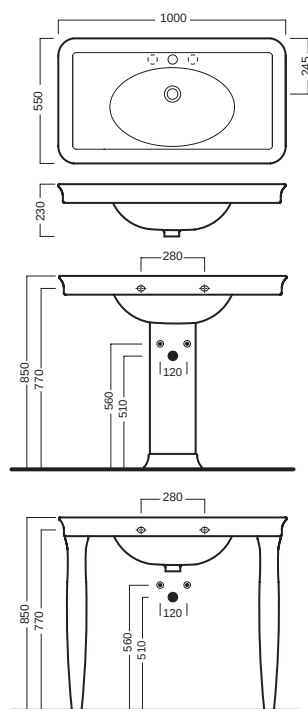
lavabo 100 washbasin 100
