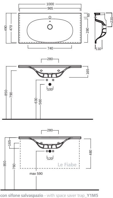
lavabo 100 washbasin 100
