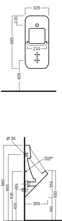
orinatoio sospeso wall hung urinal
