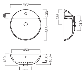
lavabo 03:00 washbasin 03:00
