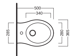
bidet sospeso_50 wall hung bidet_50
