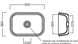
lavabo 55 washbasin 55
