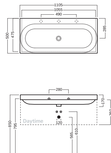
lavabo 110 washbasin 110
