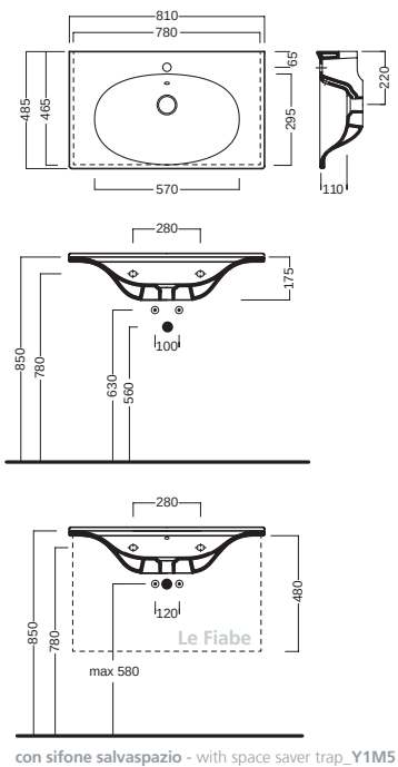
lavabo 80 washbasin 80
