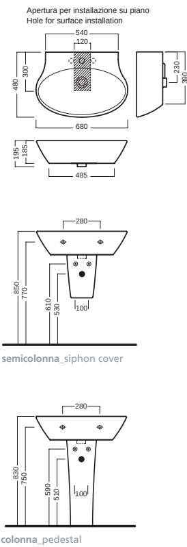
lavabo 68 washbasin 68
