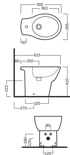
bidet bidet
