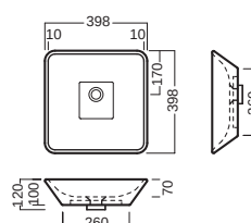
lavabo 10:00 washbasin 10:00
