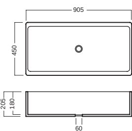
lavabo a canale 90 sink 90
