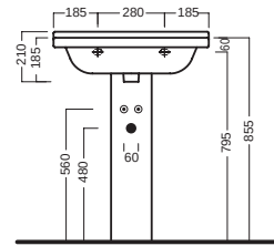
colonna_pedestal
