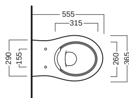
vaso filo muro PURE RIM PURE RIM back to wall wc
