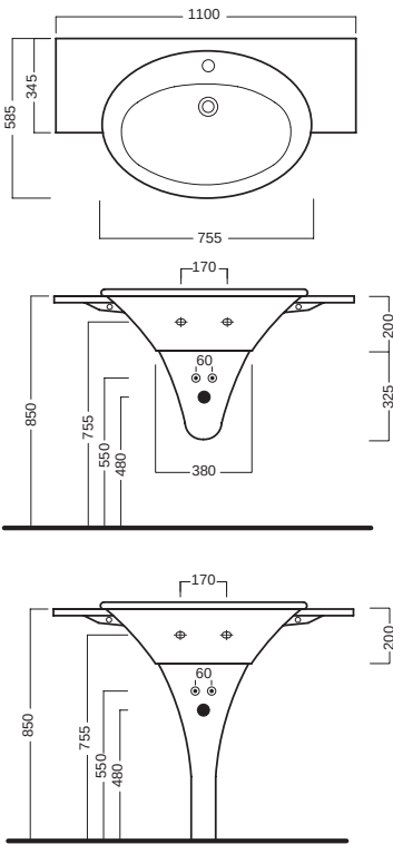
lavabo 110 washbasin 110
