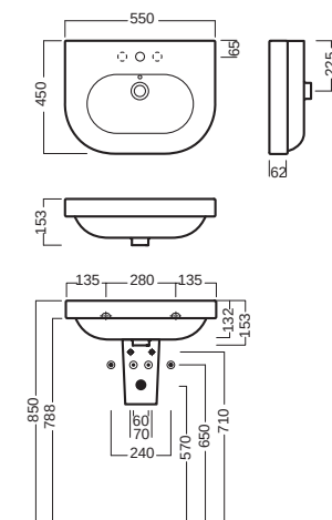
lavabo 55 washbasin 55
