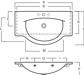
lavabi 120-105-95-86-75-56 washbasins 120-105-95-86-75-56
