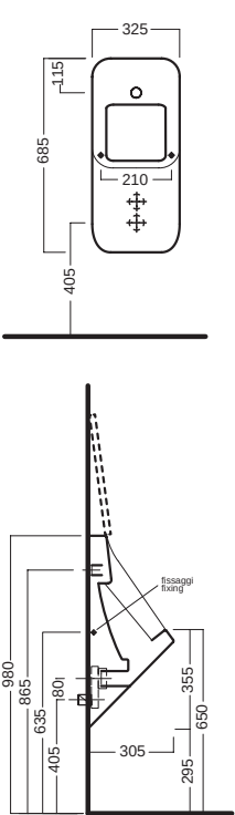
orinatoio sospeso con coperchio wall hung urinal with cover
