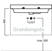
con sifone salvaspazio - with space saver trap_Y1M5
