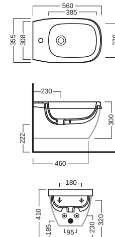
bidet sospeso wall hung bide
