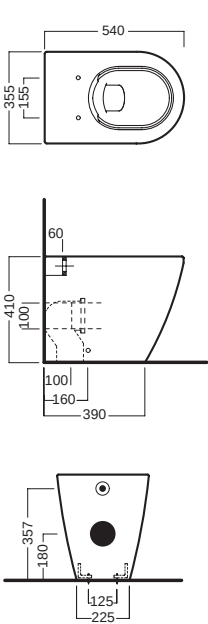
vaso filo muro PURE RIM PURE RIM back to wall wc
