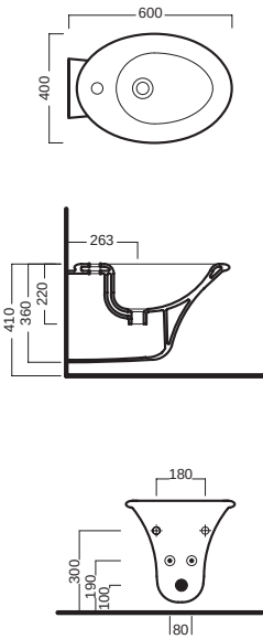
bidet sospeso wall hung bidet
