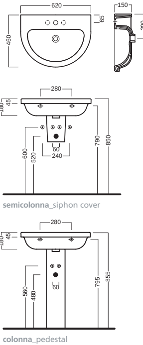
lavabo 62 washbasin 62
