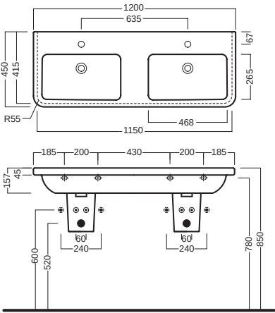
lavabo 120 washbasin 120
