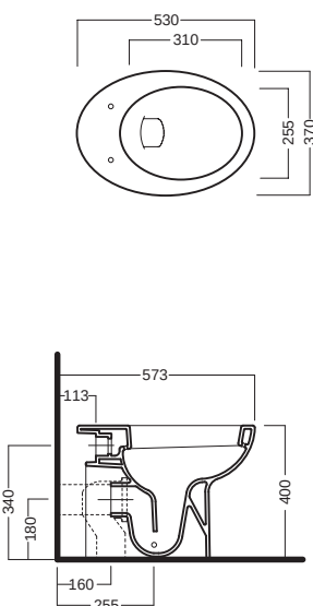
vaso wc
