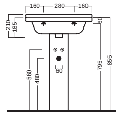
colonna_pedestal
