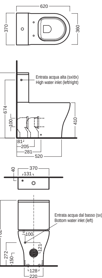
vaso PURE RIM monoblocco con cassetta PURE RIM coupled wc with cistern
