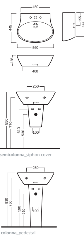
lavabo 56 washbasin 56
