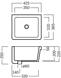
lavatoio 38 sink 38
