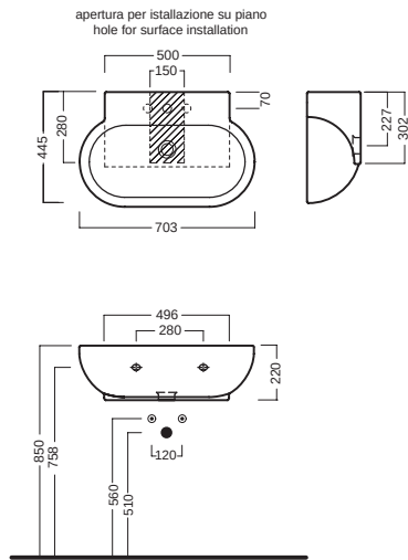
lavabo 70 washbasin 70
