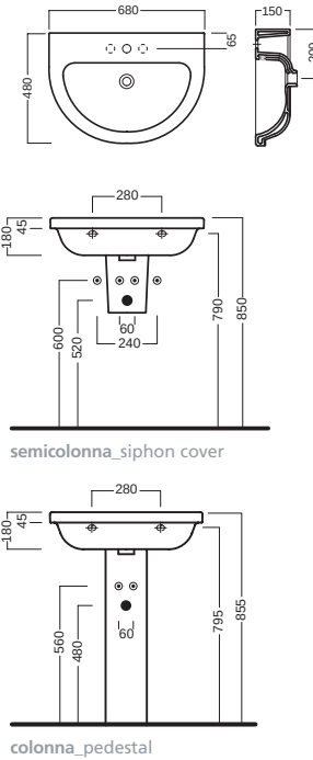
lavabo 68 washbasin 68
