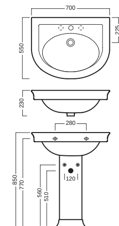
lavabo 70 washbasin 70
