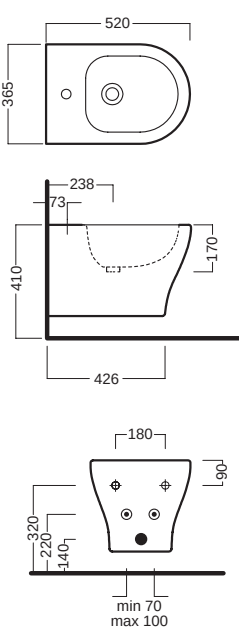
bidet sospeso wall hung bidet
