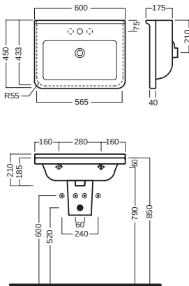
semicolonna_siphon cover
