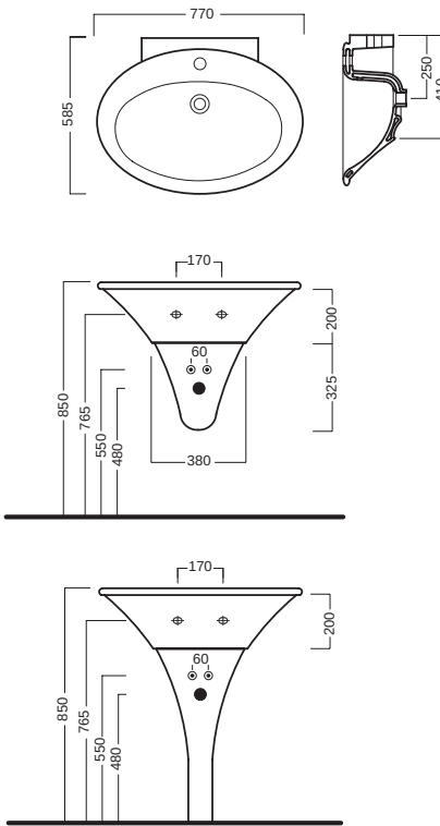
lavabo 77 washbasin 77
