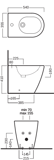
bidet filo muro back to wall bidet
