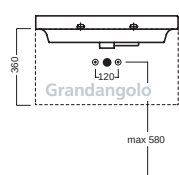
con sifone salvaspazio - with space saver trap_Y1M5
